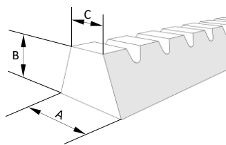
K-Profil gekerbt
